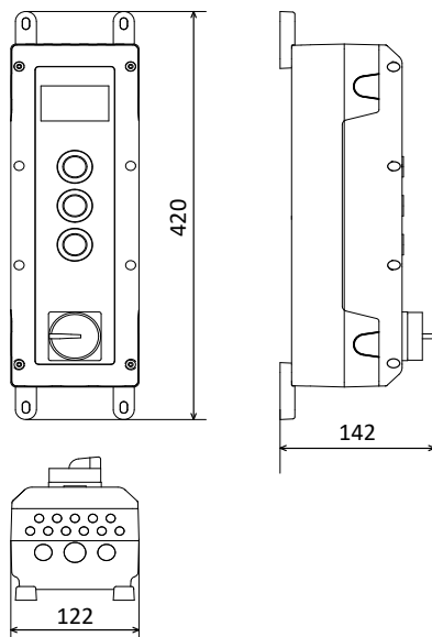
Рисунок 2. Блок управления
